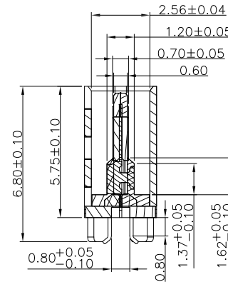
截面 A-A
